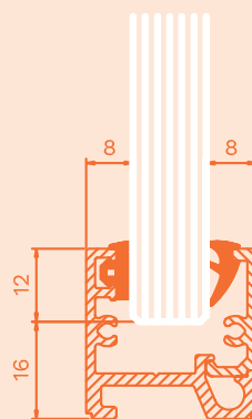
N28 med kilgummi 2, för 12-12,76 mm glas.
