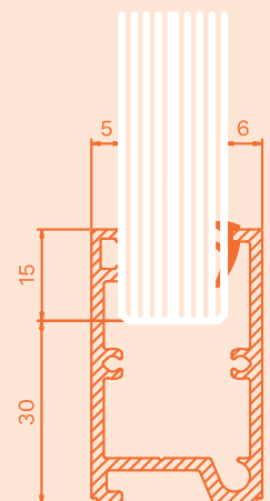
N45 med kilgummi 1, för 16,52 mm glas.
