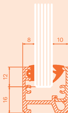
N28 med kilgummi 3, för 10-10,76 mm glas.
