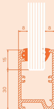
N45 med kilgummi 2, för 12-12,76 mm glas.
