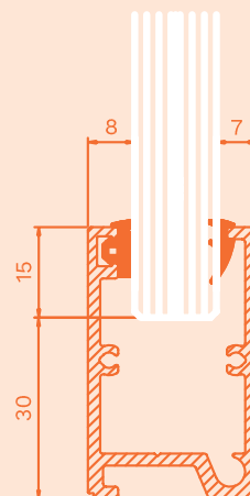
N45 med kilgummi 1, för 13,52 mm glas.
