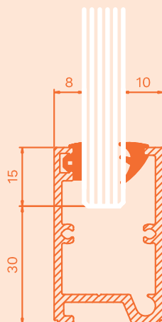
N45 med kilgummi 3, för 10-10,76 mm glas.
