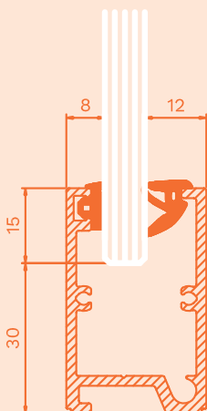
N45 med kilgummi 4, för 8-8,76 mm glas.
