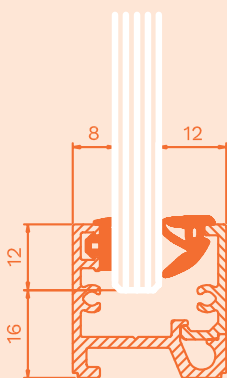
N28 med kilgummi 4, för 8-8,76 mm glas.
