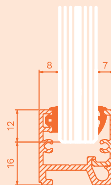
N28 med kilgummi 1, för 13,52 mm glas.
