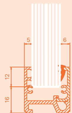
N28 med kilgummi 1, för 16,52 mm glas.
