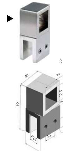
Glasbeslag justerbart 6, 8, 10 mm glas
