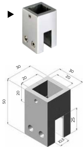
Glasbeslag Lodret stang 6, 8, 10 mm glas
