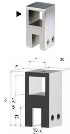
Glasbeslag Midterste/parallel 6, 8, 10 mm glas
