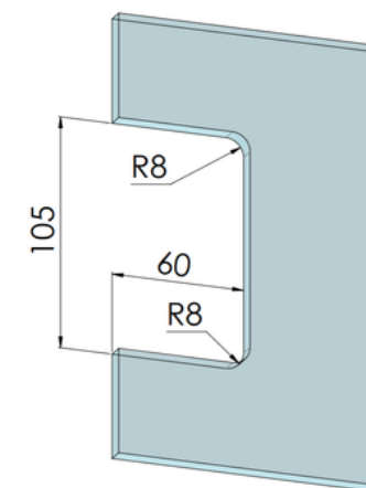
Glasudskæring GC Fenix-lås
