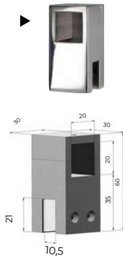
Glasbeslag Ende af rør 6, 8, 10 mm glas
