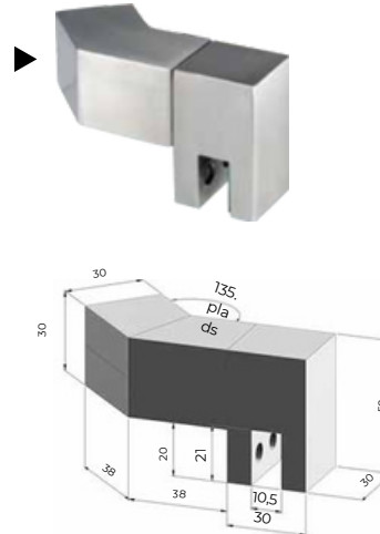
Glasbeslag 135° 6, 8, 10 mm glas
